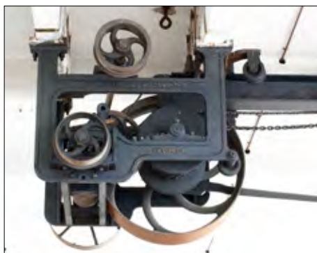
▲ Hijsinstallatie.
