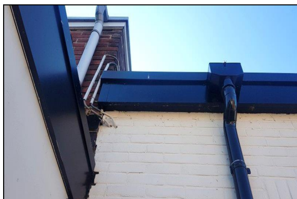
Figuur 9. Afwerking van de dakranden.
