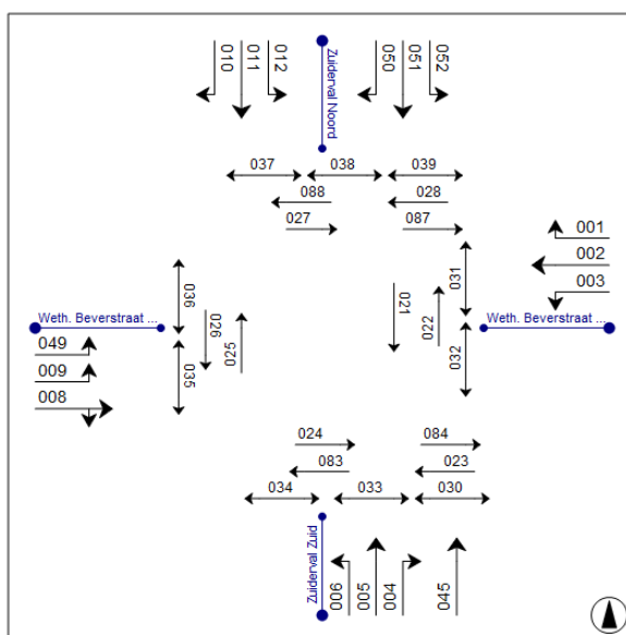
Figuur B1.1: Schema signaalgroepen kruispunt Wethouder Beverstraat - Zuiderval 5
