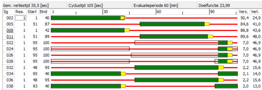
Figuur B1.5: Fasendiagram referentie Wethouder Beverstraat – Kuipersdijk
