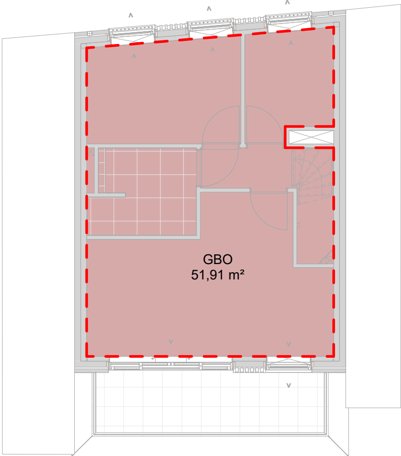
derde verdieping GBO
